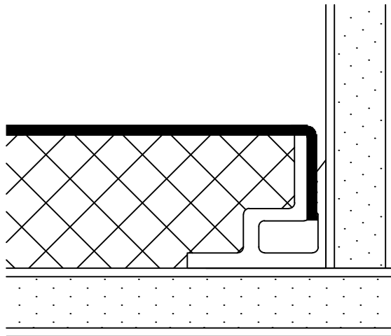
EDGE @ INSIDE CORNER
