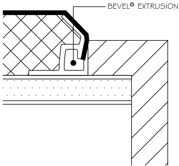
EDGE @ DOOR JAMB
