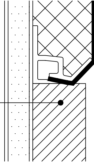
EDGE @ WOOD BASE
