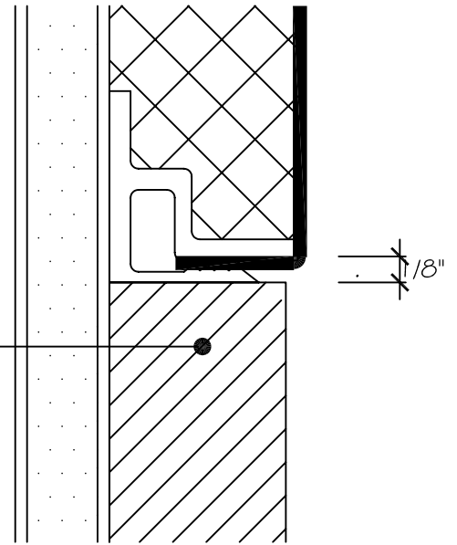
EDGE @ WOOD BASE
