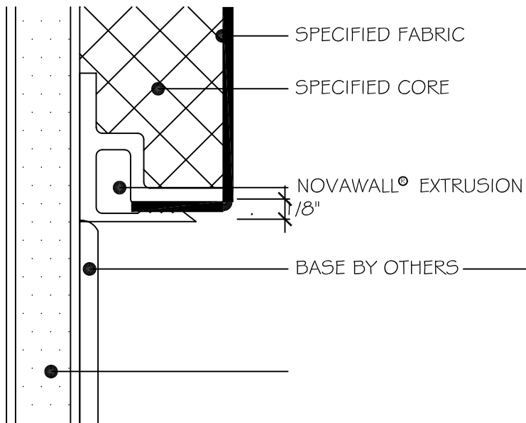
EDGE @ VINYL BASE
