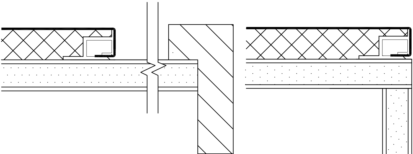
EDGE @ DOOR JAMB
