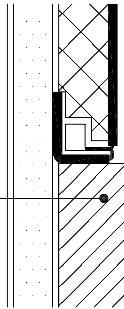
EDGE @ WOOD BASE
