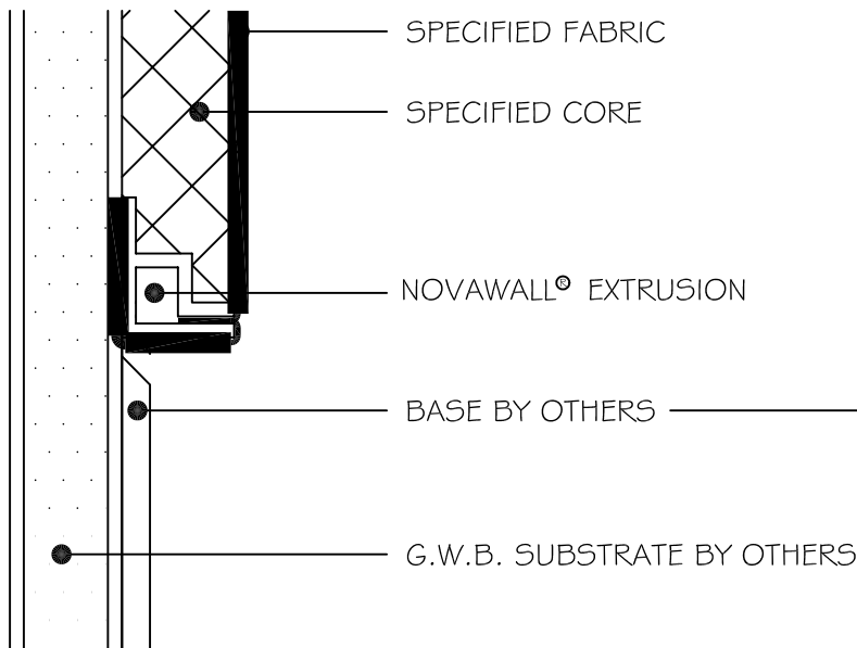
EDGE @ VINYL BASE
