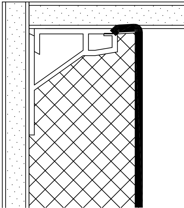
2" EDGE @ CEILING
